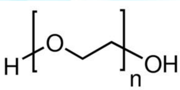
聚乙二醇
