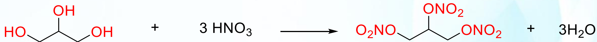
硝酸甘油
