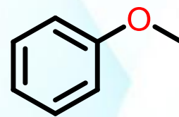
苯甲醚
